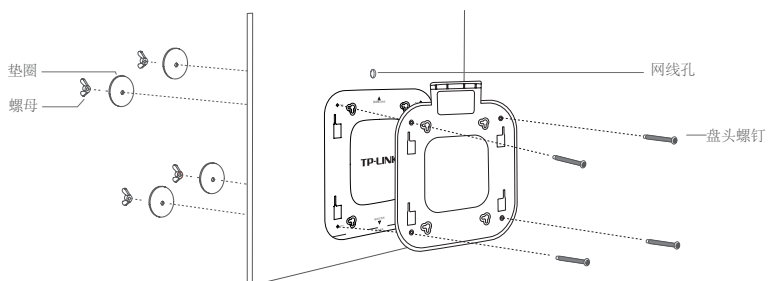
图3-4 固定安装架到天花板示意图
