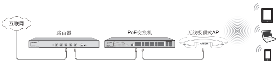
图1-4 典型应用拓扑图-FAT AP模式
