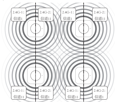
图1-3 高密度无线吸顶式AP推荐布局方式
